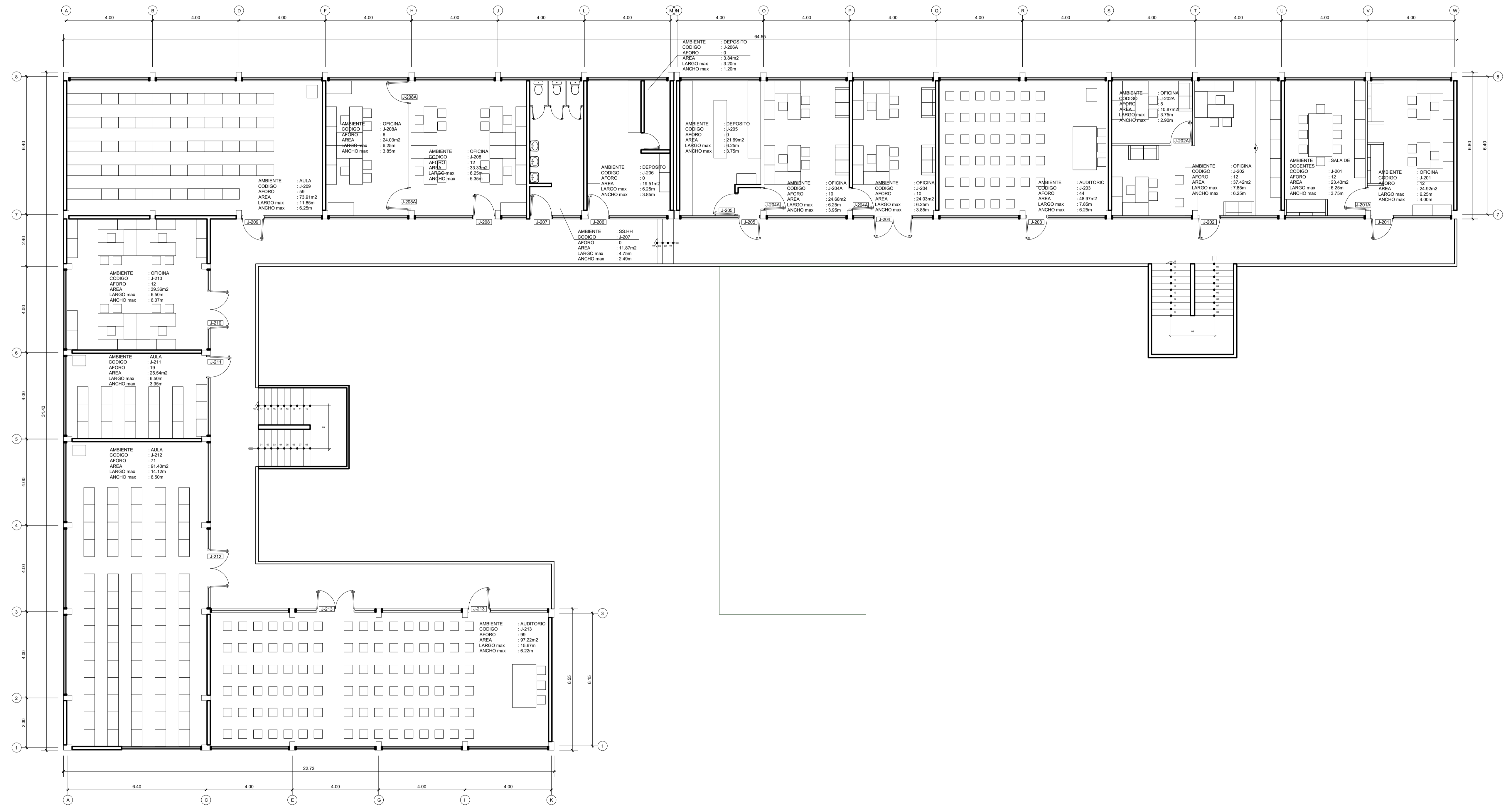
SEGUNDA PLANTA AREA TECHADA = 936.72m 2 AFORO = 383 ESCALA 1:100
